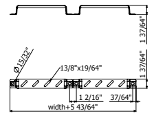
SV 16" / 20" / 24"
